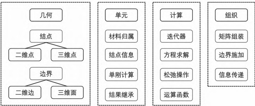
图 5 实体有限元程序设计的一些要点与功能
