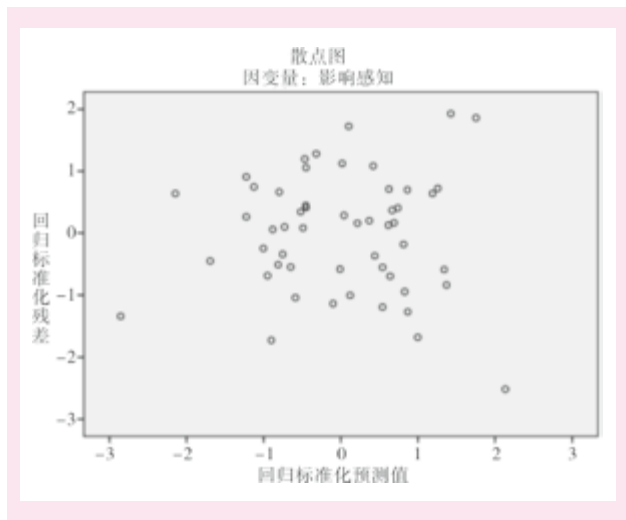
图1 标准化残差散点图
