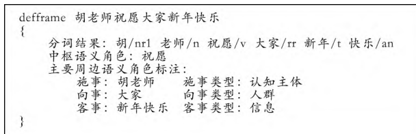
图 3 从最优解析树中产生的语义角色标注框架
