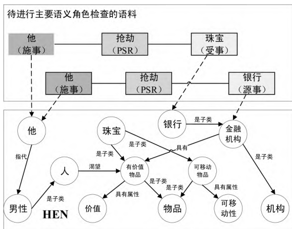
图 11 语义角色在 HEN 中被自动检查的过程
