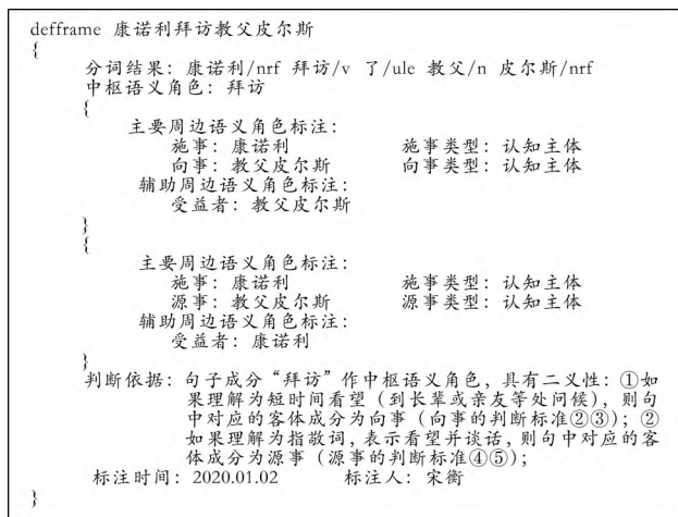
图7 中枢语义角色多义性的语义角色标注
