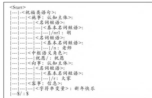
图 2 FSTD 语义文法解析得出的最优解析树
