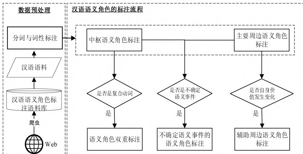
图 1 汉语语义角色的标注流程
